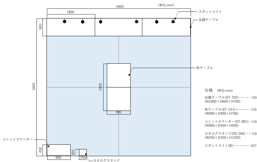
図. 基礎ブース (予定)
